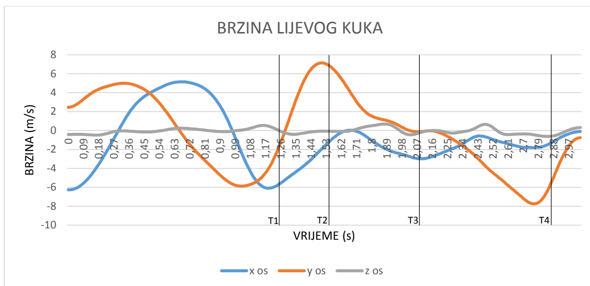
Grafički prikaz 27. Brzina lijevog kuka u tri osi
