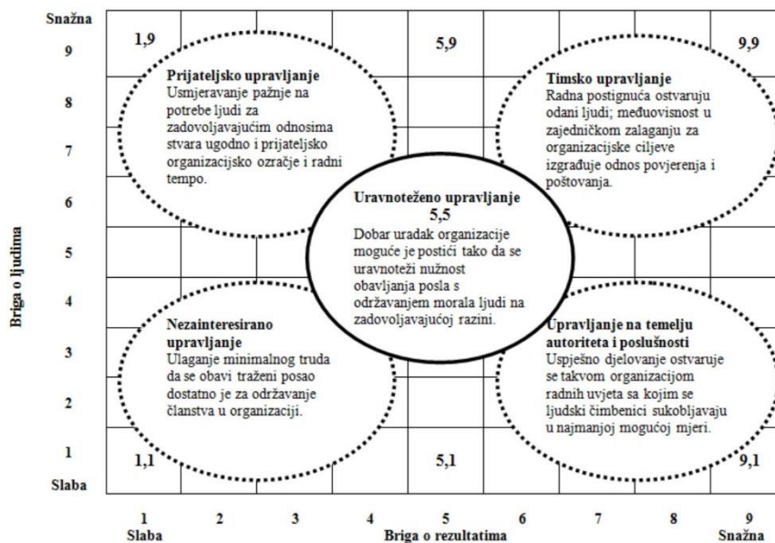
Slika 1. Mreža vodstva.
