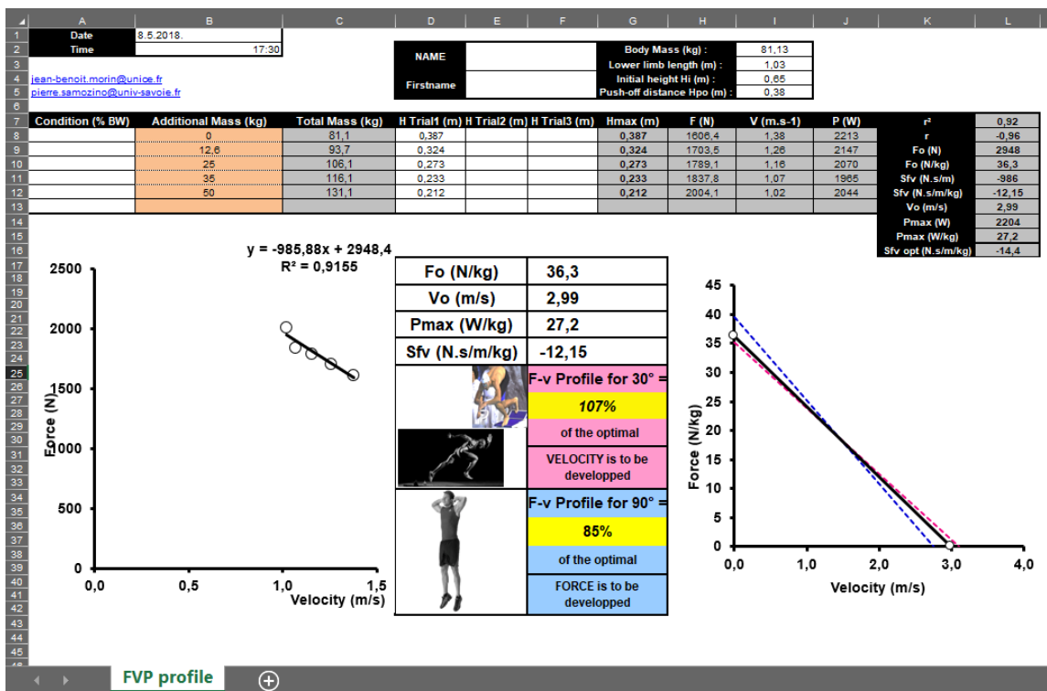
Slika 14. Prikaz proračunske tablice za izračunavanje F-v profila
