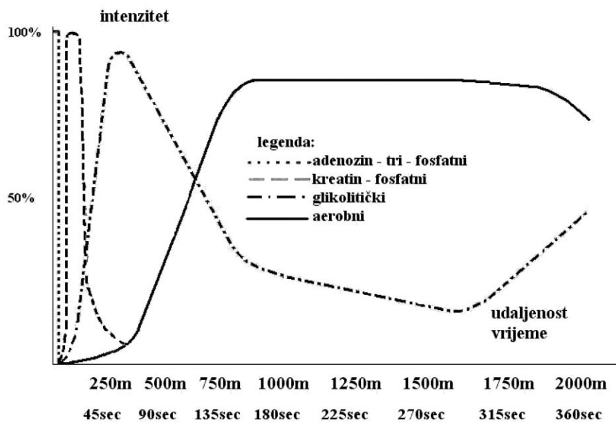
Slika 2. Grafički prikaz Dinamika energetska procesa za vrijeme veslačke utrke (Milanović, 2005, prema Bompa, 1994).
