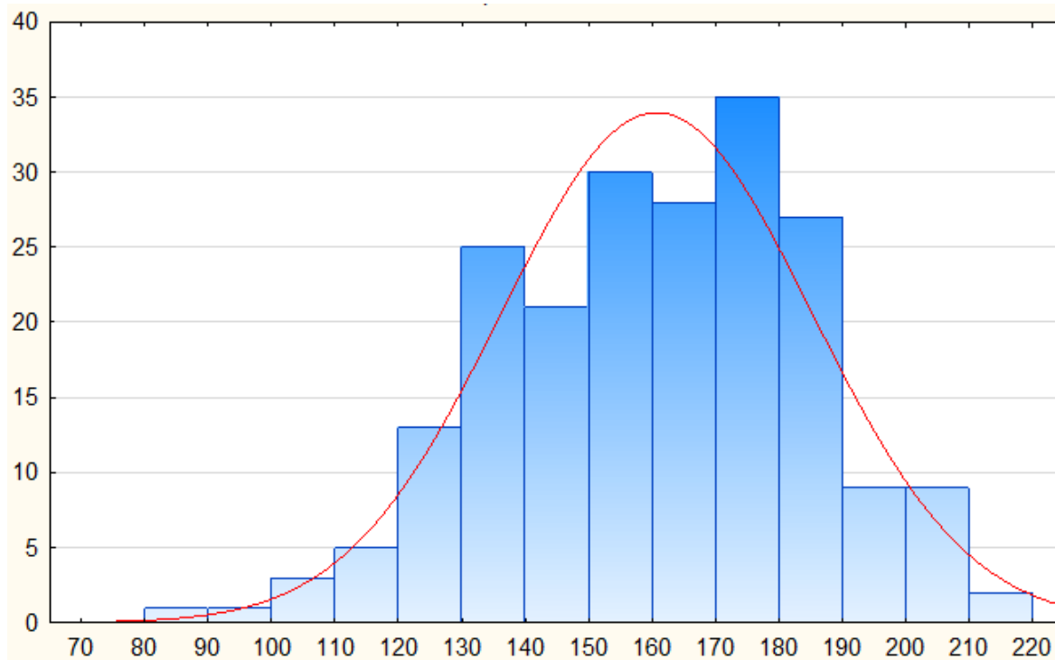
Slika 1. Histogram frekvencija ukupnog rezultata u novokonstruiranoj skali stava prema judu: na osi apscise se nalazi ukupni rezultat, a na osi ordinate frekvencije. Punom linijom označena je teoretska normalna distribucija.
